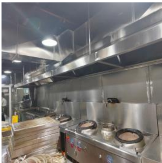
烟罩施工中
